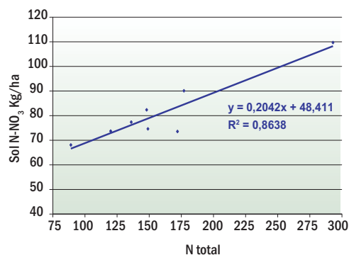
Figure 4. Relation entre la teneur en nitrates résiduels des sols après la récolte de la pomme de terre et la quantité d'azote total appliqué.
