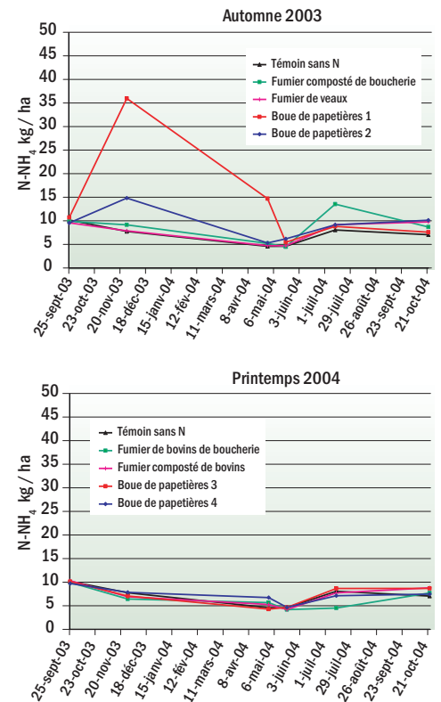
Figure 2. Quantité d'azote ammoniacal (N-NH 4 ) dans la couche de sol 0-60 cm suite aux apports d'engrais organiques effectués à l'automne 2003 et au printemps 2004.
