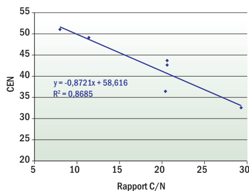
Figure 1. Relation entre le coefficient d'efficacité de l'azote (CEN) de première année des boues de papetières et des fumiers frais de bovins selon leur rapport C/N.
