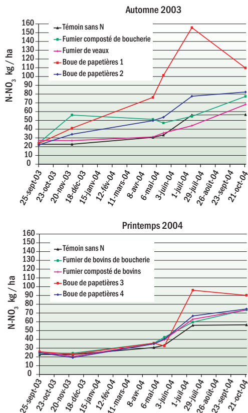
Figure 3. Quantité de nitrates ( \text{N-NO}_3 ) dans la couche de sol 0-60 cm suite aux apports d'engrais organiques effectués à l'automne 2003 et au printemps 2004.
